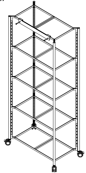
PIXEL RACK M 820x460,5x1935 mm mit PIXEL Whiteboard Halterung. with PIXEL whiteboard holder.
