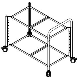
PIXEL RACK M 820x460,5x564 mm mit Griffbügel. with PIXEL Rack Handle.
