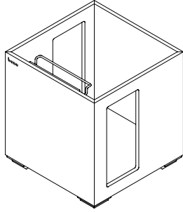
PIXEL BOX MIT SEITLICHEN ÖFFNUNGEN PIXEL BOX WITH OPENINGS ON THE SIDE 360x360x381 mm
